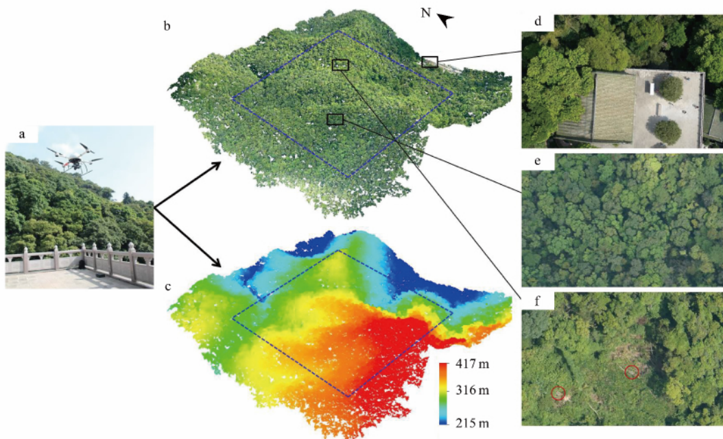
图 3 基于一个 20 公顷常绿阔叶林样地的无人机调查(引自: Zhang 等 [25] )
