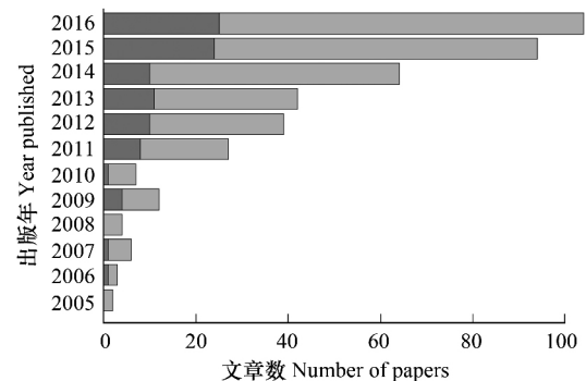
图2 基于 ISI Web of Science 的无人机遥感相关论文数量统计
